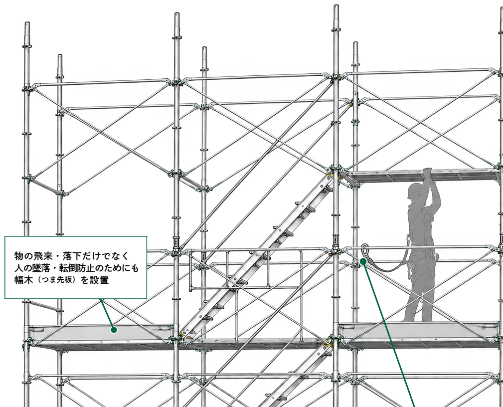
わく組足場
